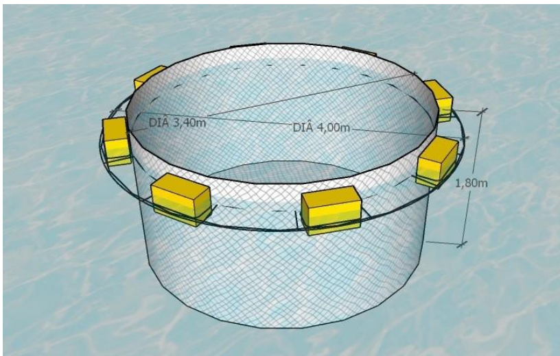
Figura 4 – Desenho esquemático da unidade de produção, tanque-rede cilíndrico em varão de aço galvanizado com malha trançada em aço inox apoiado sobre flutuantes plásticos ( \text{Ø}3,4 \times 1,6 \text{ m} ).
